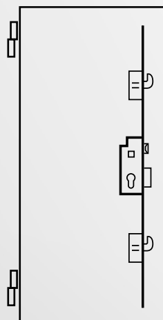
2 hooks art. 2815201354 art. 2845201354
