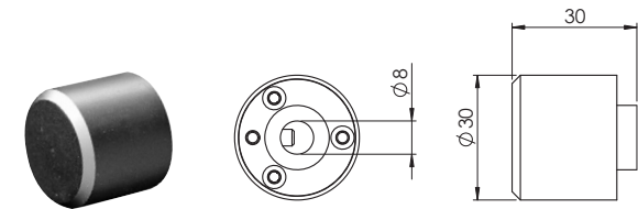
ANTI BARRICADE KNOB
